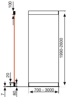
COMET SABİT ALT VE ÜST BAZA
